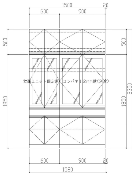
展開A図
