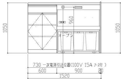
展開A図
